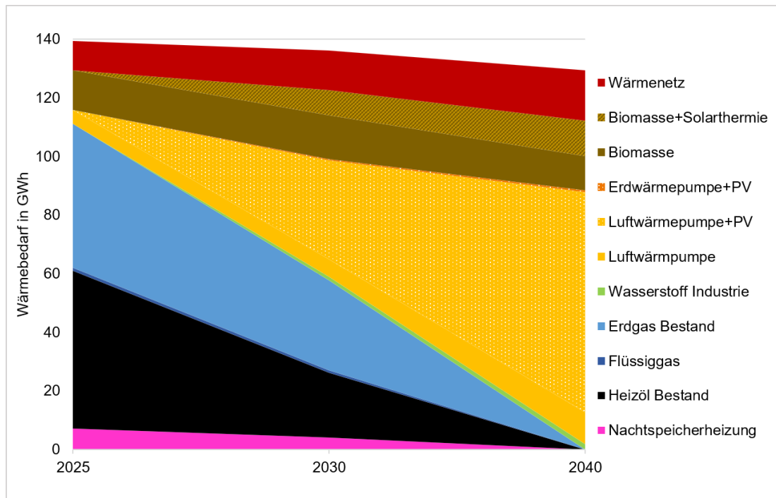
Abbildung 49: Transformation der Wärmebereitstellung im MIX-Szenario
