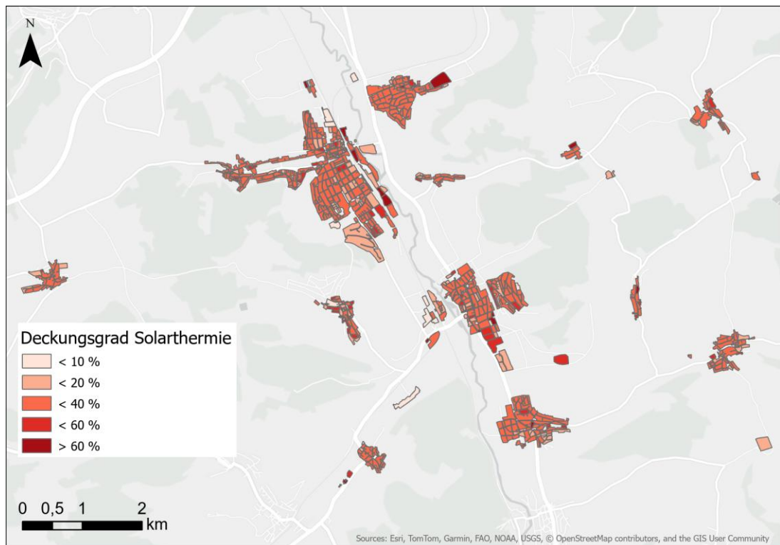
Abbildung 27: Kartografische Darstellung des potenziellen Deckungsgrads von Solarthermie-Anlagen
