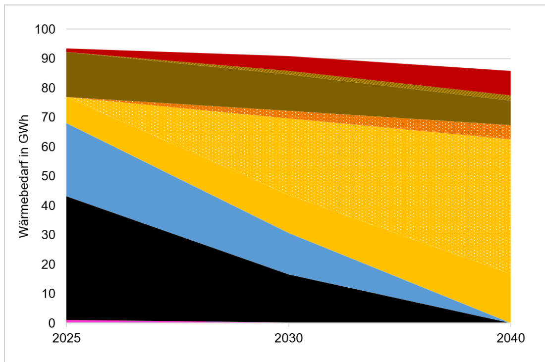
Abbildung 47: Transformation der Wärmebereitstellung im WÄRMENETZE-Szenario
