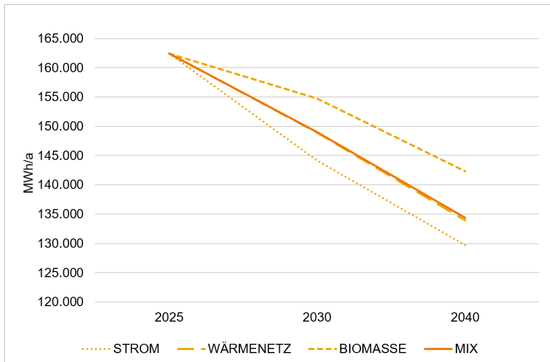
Abbildung 50: Entwicklung des Endenergiebedarfs in den berechneten Szenarien
