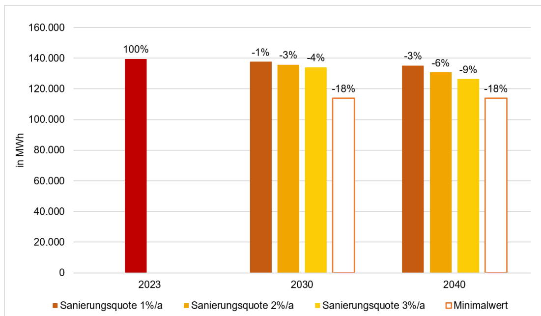
Abbildung 19: Wärmebedarfsreduktion durch Sanierung Wohnen
