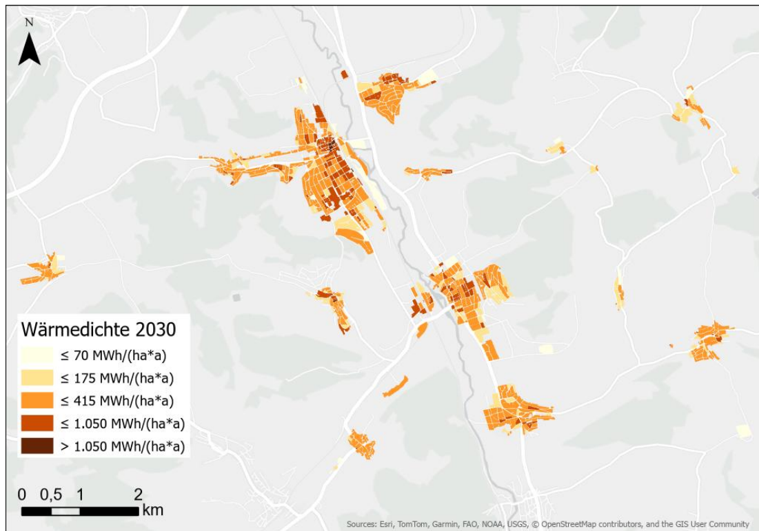
Abbildung 36: Wärmedichten im Jahr 2030
