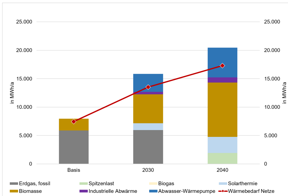
Abbildung 55: Möglicher Energiemix in den zukünftigen Wärmenetzen
