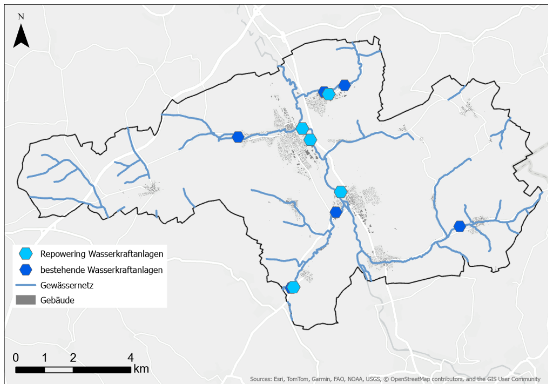
Abbildung 29: Potenzial Wasserkraftanlagen Lauda-Königshofen
