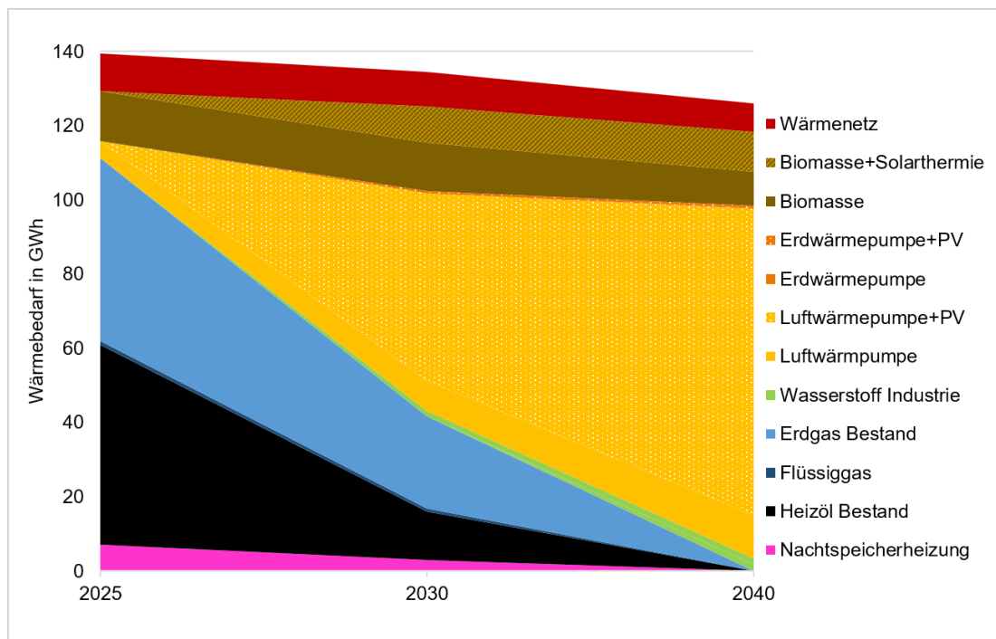
Abbildung 46: Transformation der Wärmebereitstellung im STROMNETZ-Szenario
