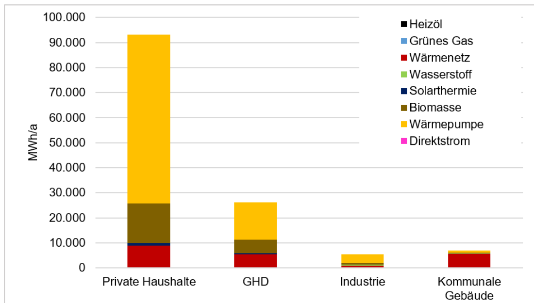
Abbildung 54: Wärmebedarf im Jahr 2040 nach Sektoren und Energieträgern
