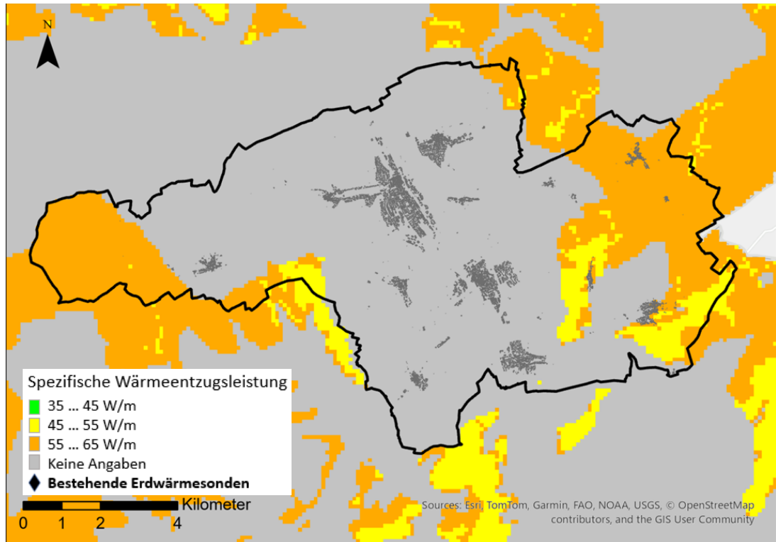
Abbildung 30: Darstellung der spezifischen Wärmeentzugsleistung (100 m, 1.800 h/a)
