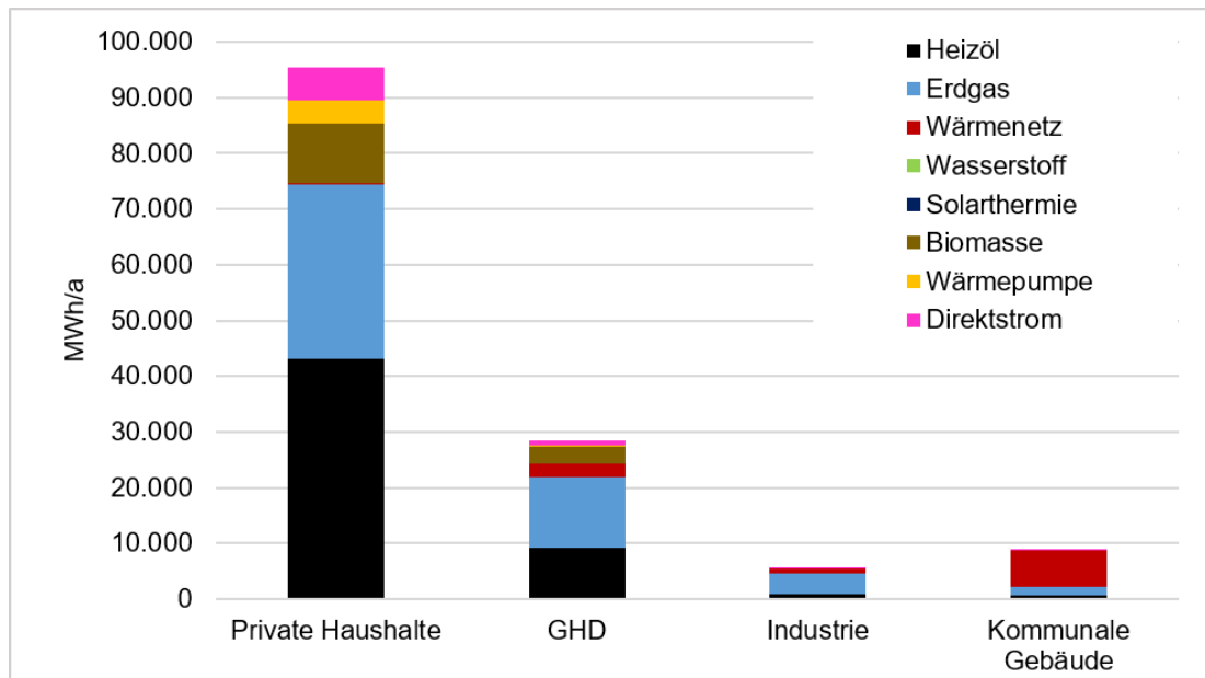
Abbildung 52: Wärmebedarf im Basisjahr 2023 nach Sektoren und Energieträgern
