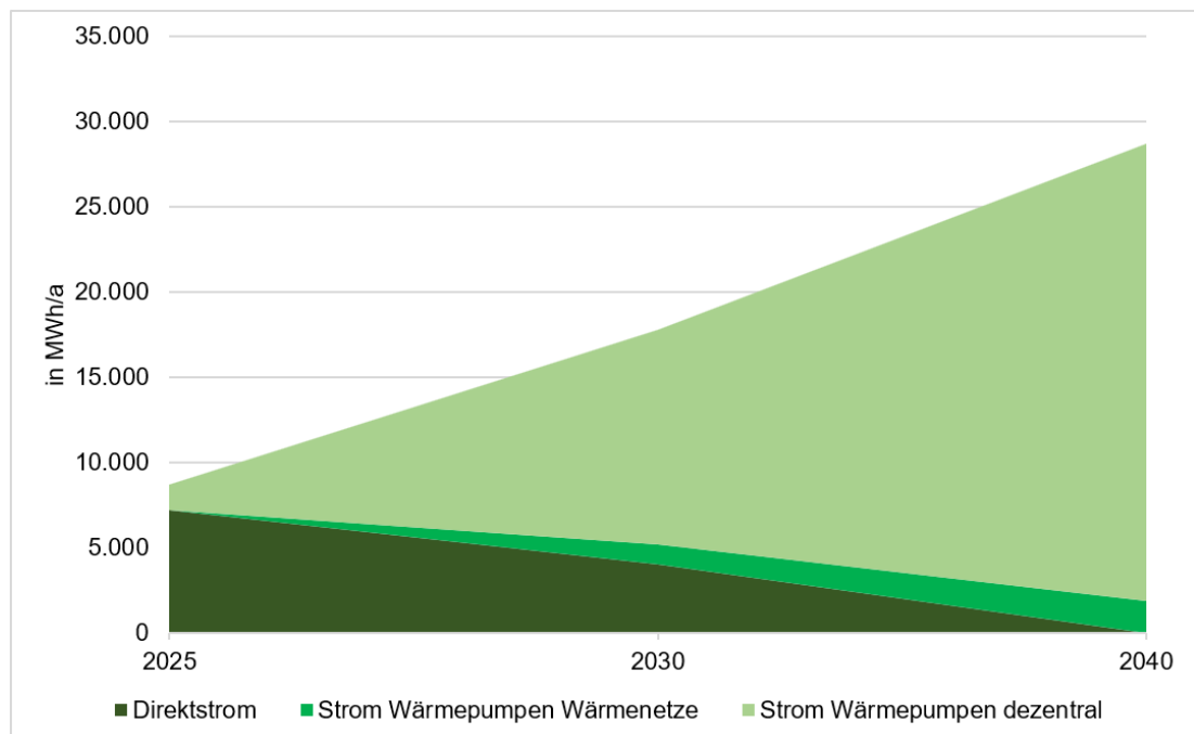
Abbildung 58: Zunahme des Strombedarfs durch Wärmerzeuger im Zielszenario
