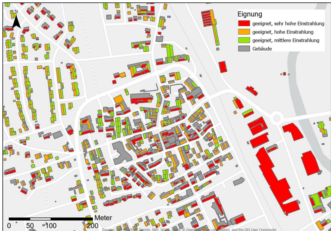
Abbildung 25: Kartografischer Ausschnitt des PV-Potenzial auf Dachflächen
