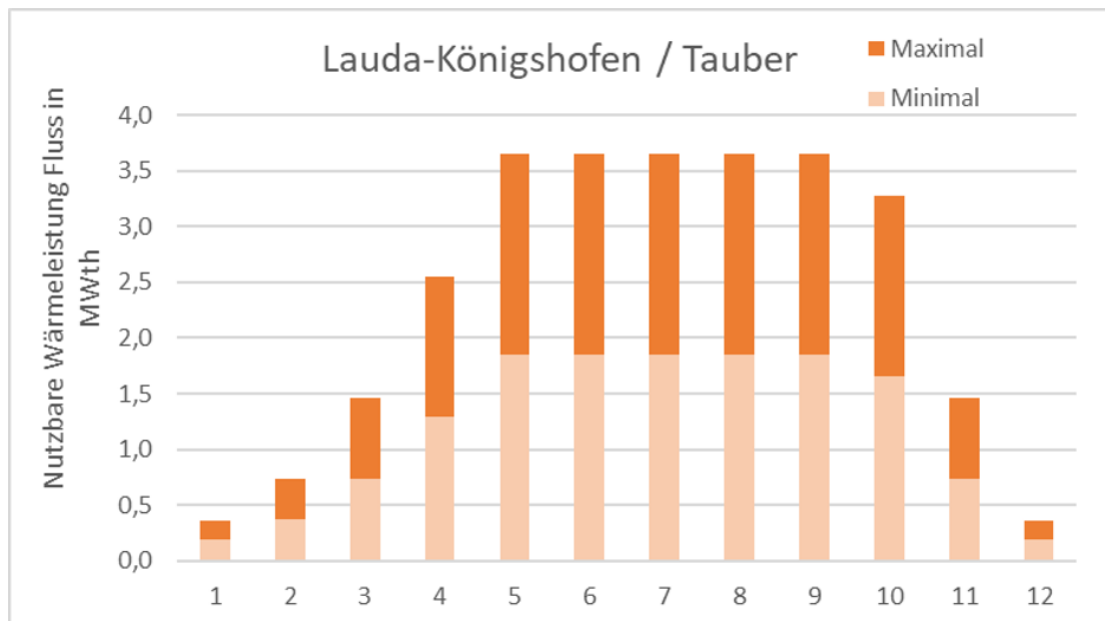
Abbildung 24: Potenzialabschätzung nutzbare Wärmeleistung Fließgewässer Tauber
