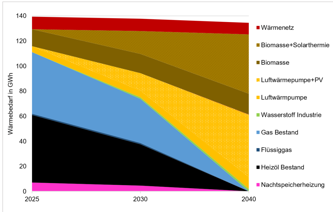
Abbildung 48: Transformation der Wärmebereitstellung im BIOMASSE-Szenario
