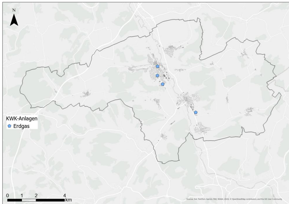
Abbildung 11: Kartografische Darstellung der bestehenden KWK-Anlagen
