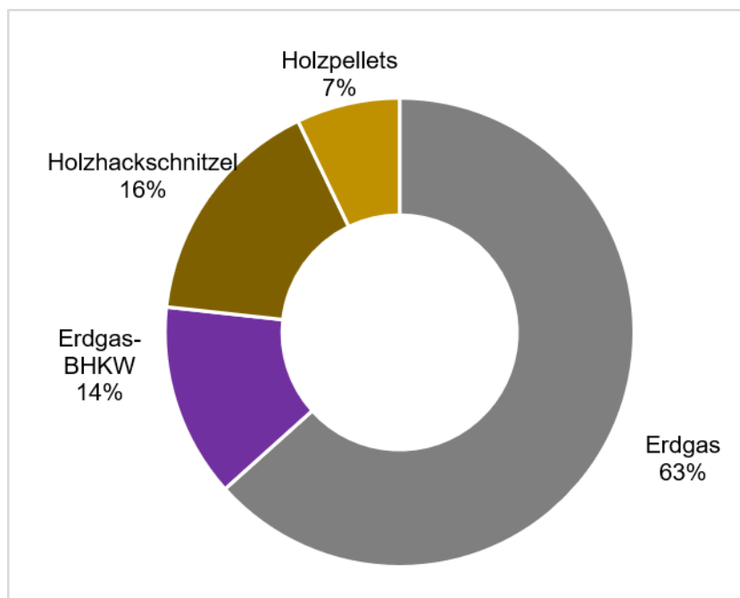
Abbildung 10: Wärmebereitstellung nach Energieträger/Technologie in den Wärmenetzen
