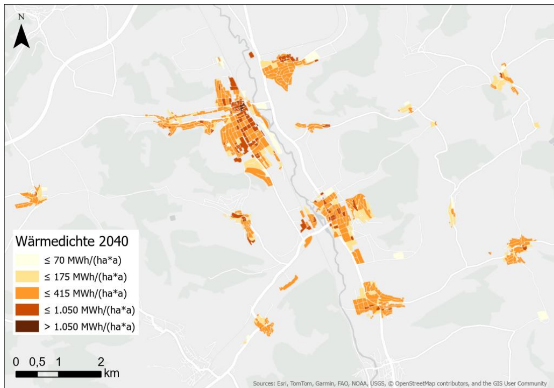
Abbildung 37: Wärmedichten im Jahr 2040
